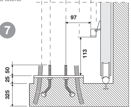
ANCLAJE Vista lateral
