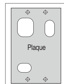
ANCORAGE DU MOTORÉDUCTEUR vue en plan
