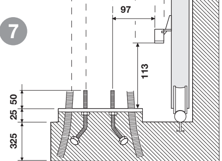
ANCORAGE DU MOTORÉDUCTEUR vue latérale
